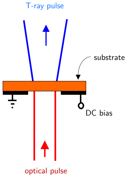
(a) PCA emitter
